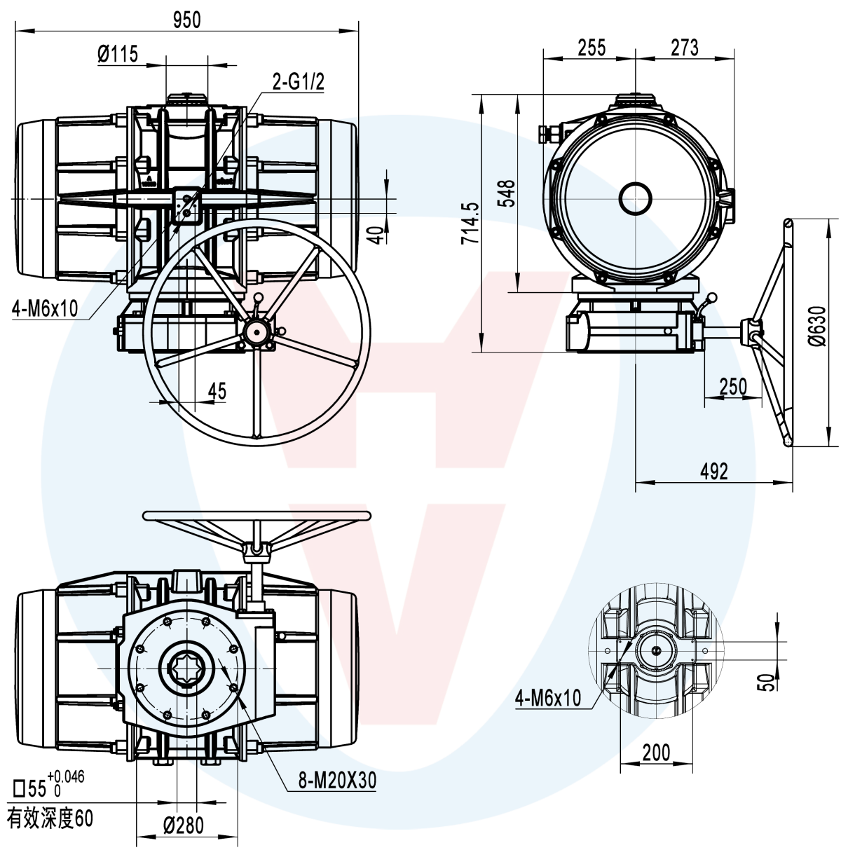
阀门连接尺寸
