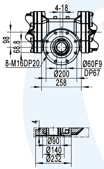
底部阀门连接尺寸
