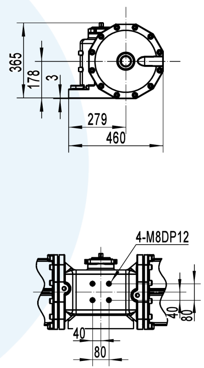
侧面连接尺寸
