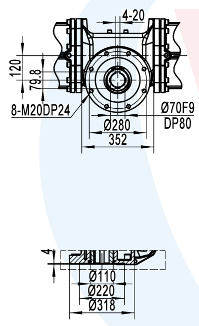
底部阀门连接尺寸
