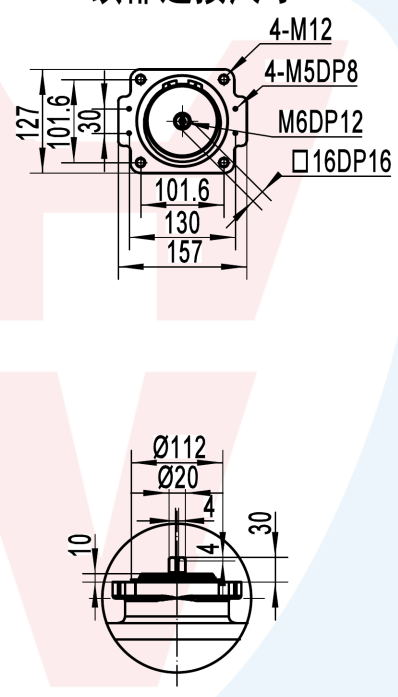
顶部连接尺寸
