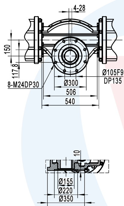
底部阀门连接尺寸
