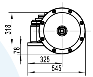
侧面连接尺寸
