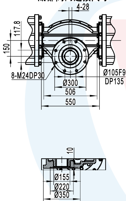
底部阀门连接尺寸
