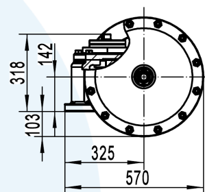
侧面连接尺寸
