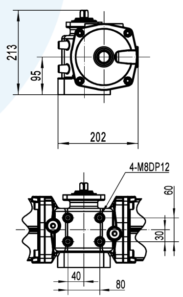
侧面连接尺寸
