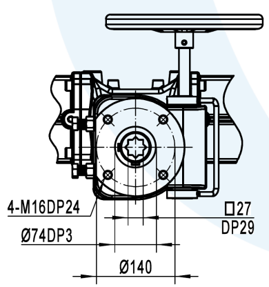
底部阀门连接尺寸
