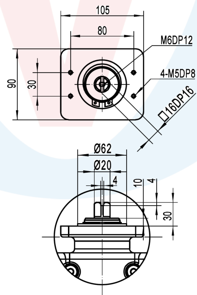
顶部连接尺寸
