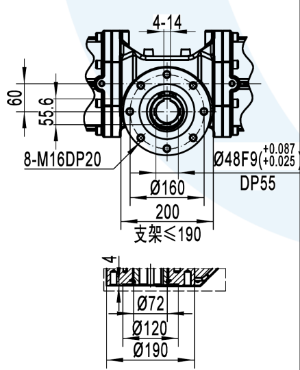
底部阀门连接尺寸
