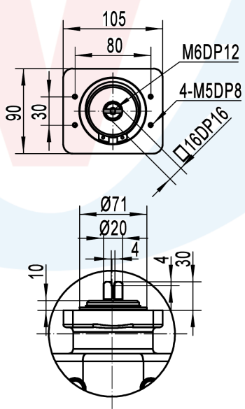
顶部连接尺寸
