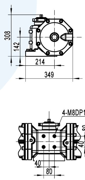
侧面连接尺寸
