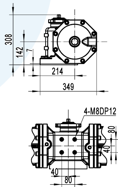
侧面连接尺寸
