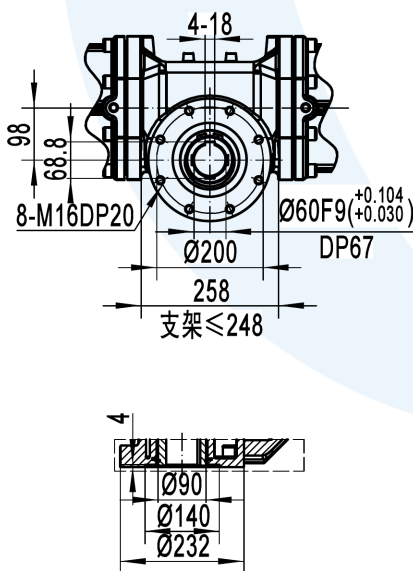
底部阀门连接尺寸
