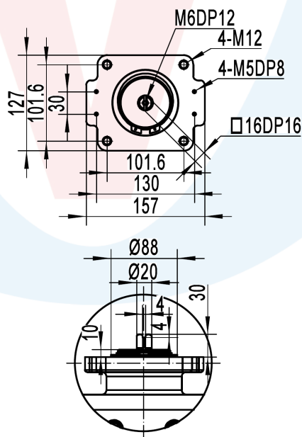
顶部连接尺寸
