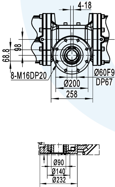
安装连接尺寸 底部阀门连接尺寸
