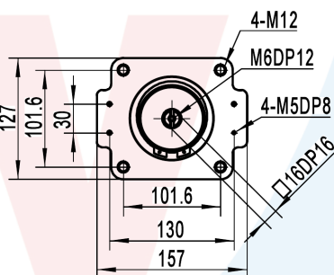
顶部连接尺寸
