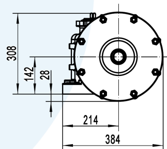
侧面连接尺寸
