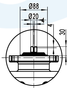
外形图
