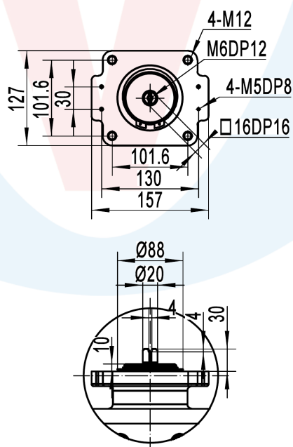
外形图
