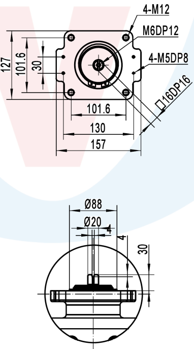
顶部连接尺寸
