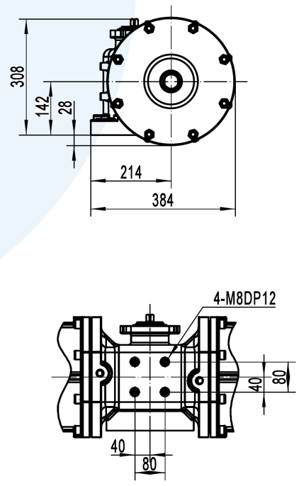
侧面连接尺寸
