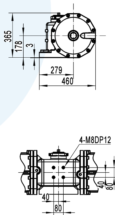
侧面连接尺寸
