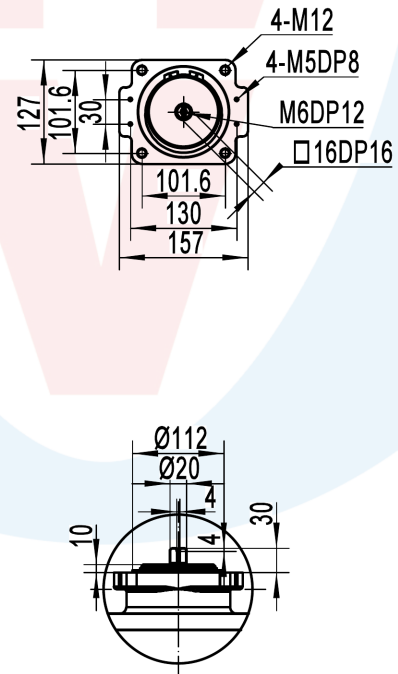
顶部连接尺寸
