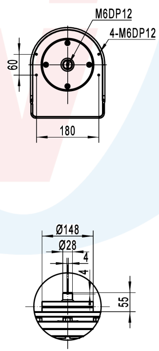
顶部连接尺寸
