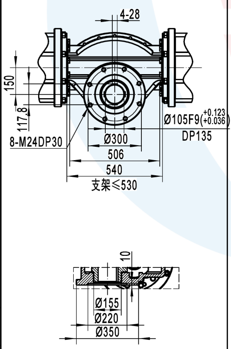
底部阀门连接尺寸
