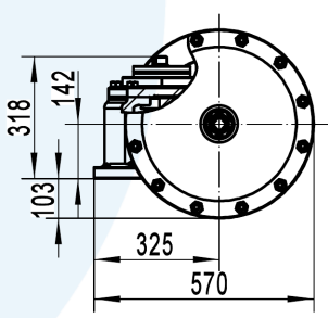
侧面连接尺寸
