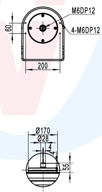
顶部连接尺寸
