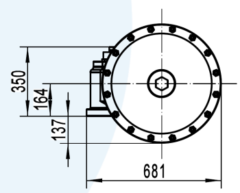
侧面连接尺寸
