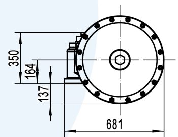
侧面连接尺寸
