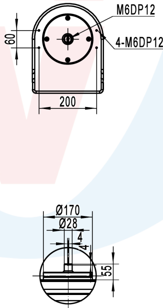
顶部连接尺寸
