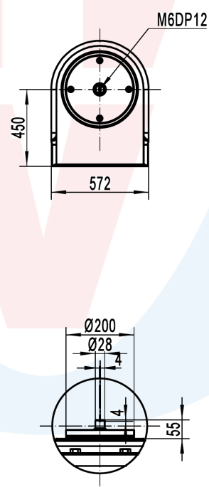
顶部连接尺寸
