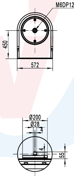
顶部连接尺寸
