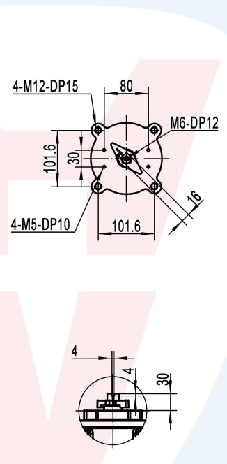
顶部连接尺寸
