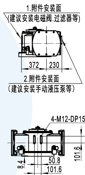
侧面连接尺寸
