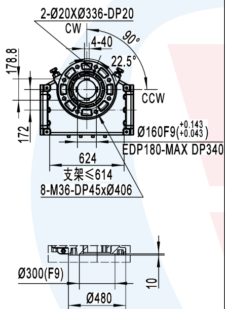
底部阀门连接尺寸
