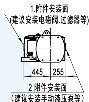
侧面连接尺寸
