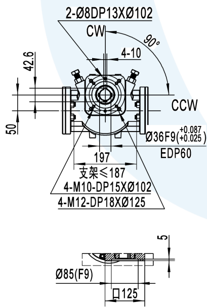
底部阀门连接尺寸
