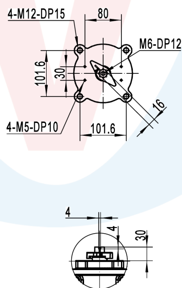
顶部连接尺寸
