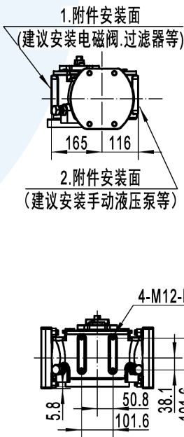
侧面连接尺寸
