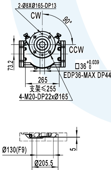
底部阀门连接尺寸
