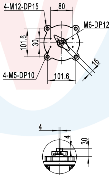
顶部连接尺寸
