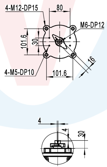
顶部连接尺寸
