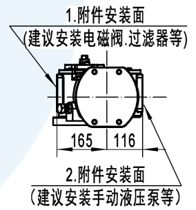
侧面连接尺寸
