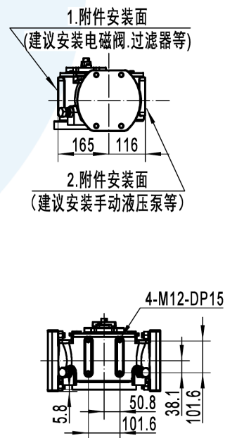
侧面连接尺寸
