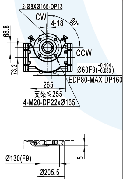
底部阀门连接尺寸
