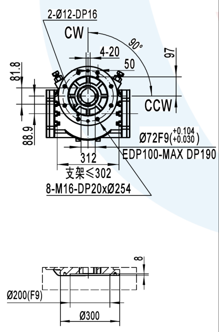
底部阀门连接尺寸
