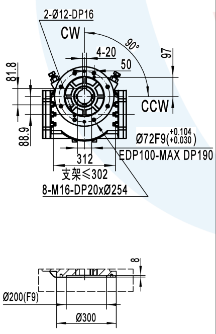
底部阀门连接尺寸
