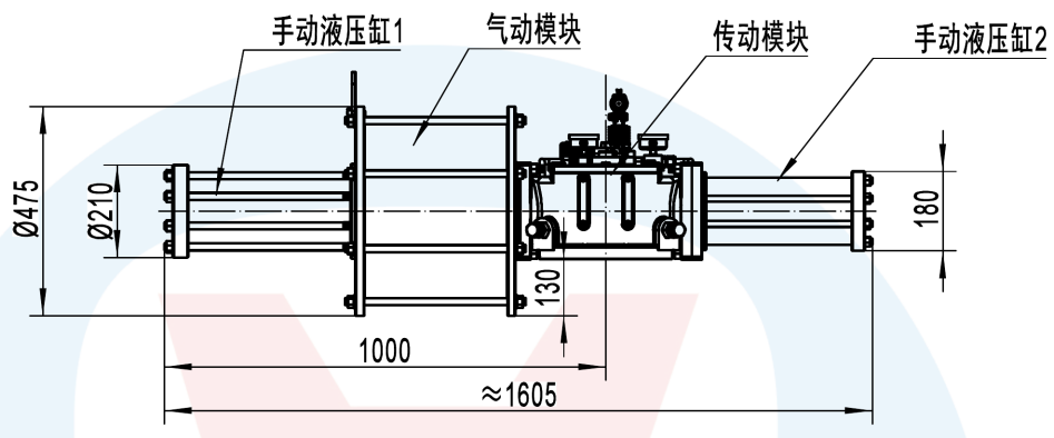
附件安装尺寸-更新日期260130
