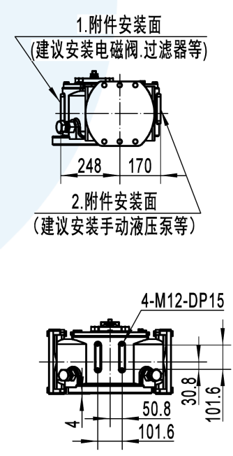
侧面连接尺寸
