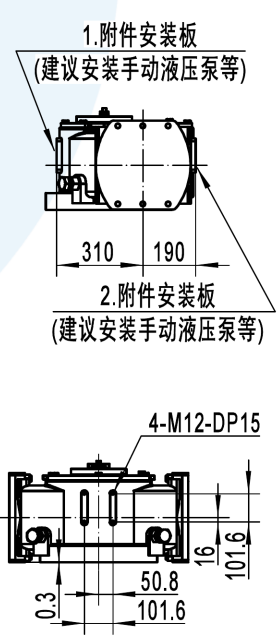
侧面连接尺寸
