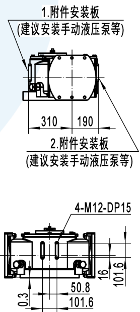
侧面连接尺寸
