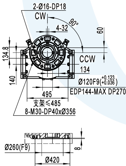
底部阀门连接尺寸
