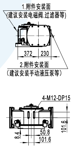
侧面连接尺寸
