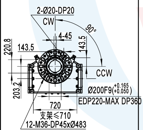
底部阀门连接尺寸
