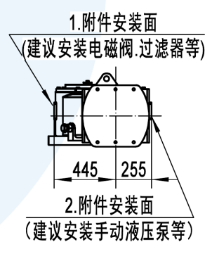
侧面连接尺寸
