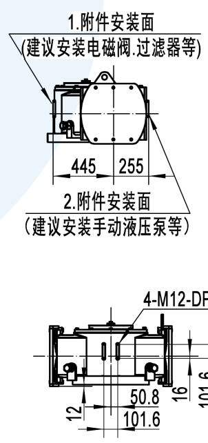
侧面连接尺寸
