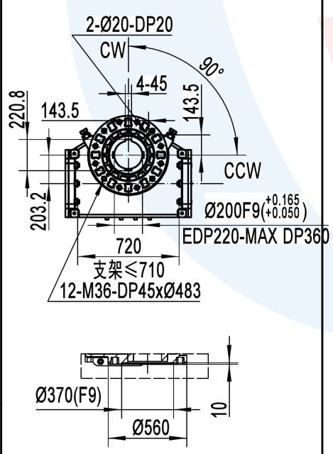
底部阀门连接尺寸
