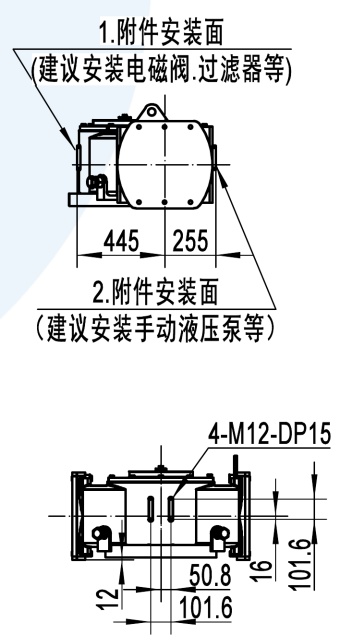
侧面连接尺寸
