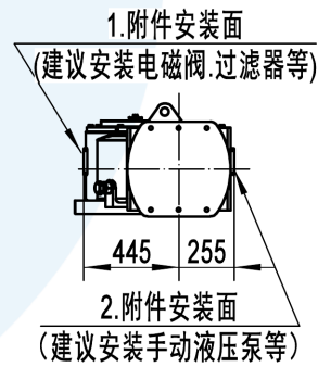
侧面连接尺寸
