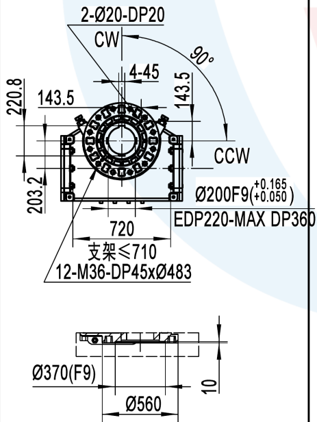
底部阀门连接尺寸
